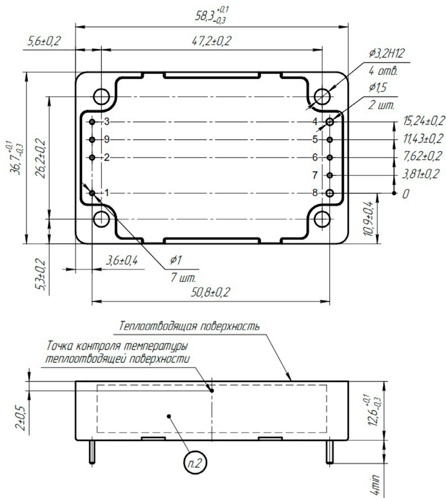
Рис. 20. Исполнение МДМ200-С.
