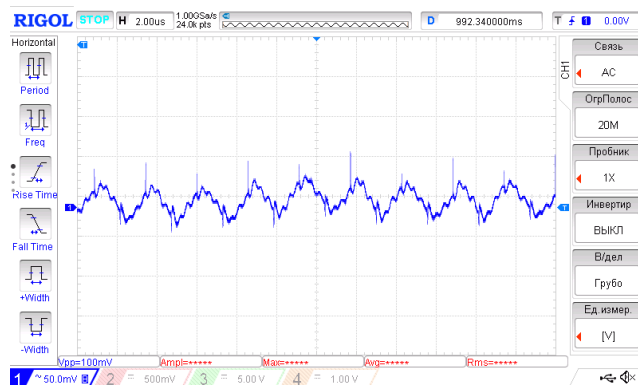
Рис. 19. Осциллограмма пульсаций U_{вых,ном} . Масштаб 50 мВ/дел. Развертка 2 мкс/дел.
