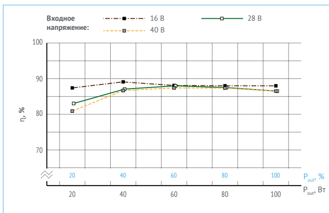
Рис. 14. МДМ200-1В15РС.
