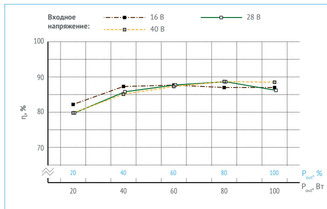
Рис. 15. МДМ200-1В24РС.
