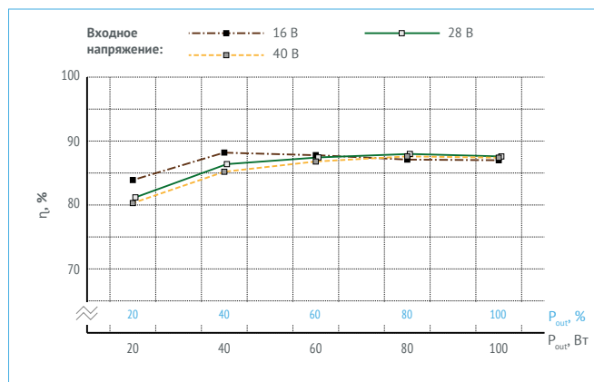
Рис. 16. МДМ200-1В27РС.
