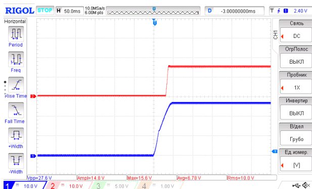
Рис. 18. Установление U_{вых,ном} с момента подачи U_{вх,ном} . Луч 1 (синий) — входное напряжение. Масштаб 10 В/дел. Луч 2 (красный) — выходное напряжение. Масштаб 10 В/дел. Развертка 50 мс/дел.
