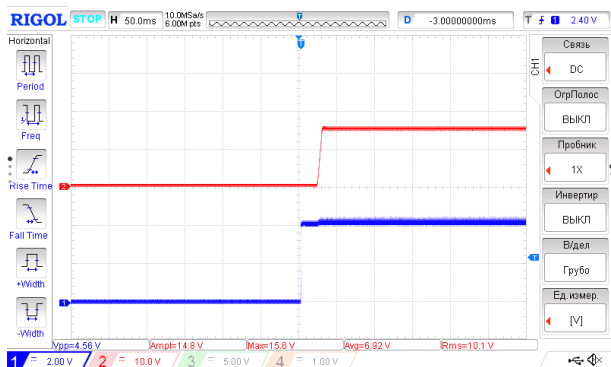
Рис. 17. Установление U_{вых,ном} с момента подачи сигнала ДУ (размыкание выводов «ДУ» и «-ВХ»). Луч 1 (синий) — напряжение на выводе «ДУ». Масштаб 2 В/дел. Луч 2 (красный) — выходное напряжение. Масштаб 10 В/дел. Развертка 50 мс/дел.
