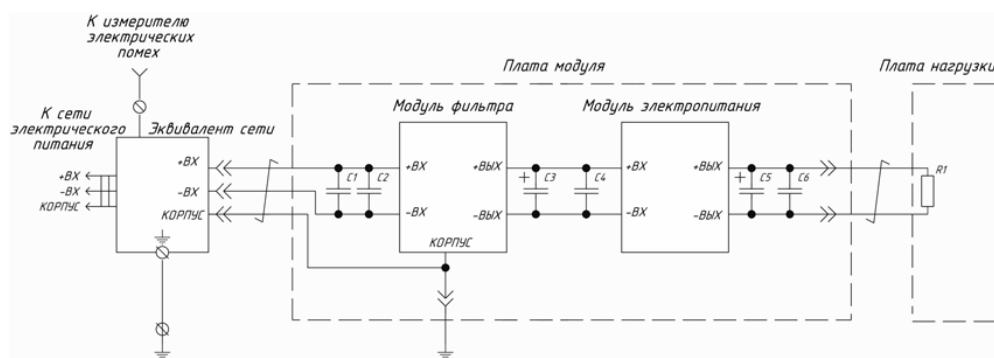
Рис. 3. Схема измерения ЭМС МДМ200-С.
