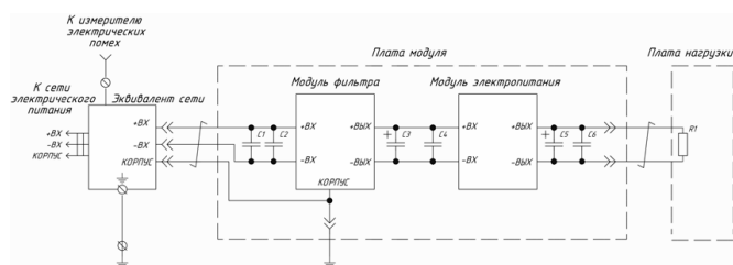
Рис. 3. Схема измерения ЭМС МДМ200-С.
