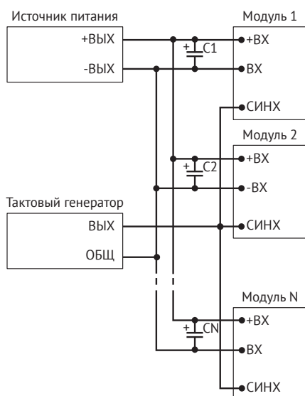
Рис. 10. Привет построения системы с синхронизацией от внешнего тактового генератора.
