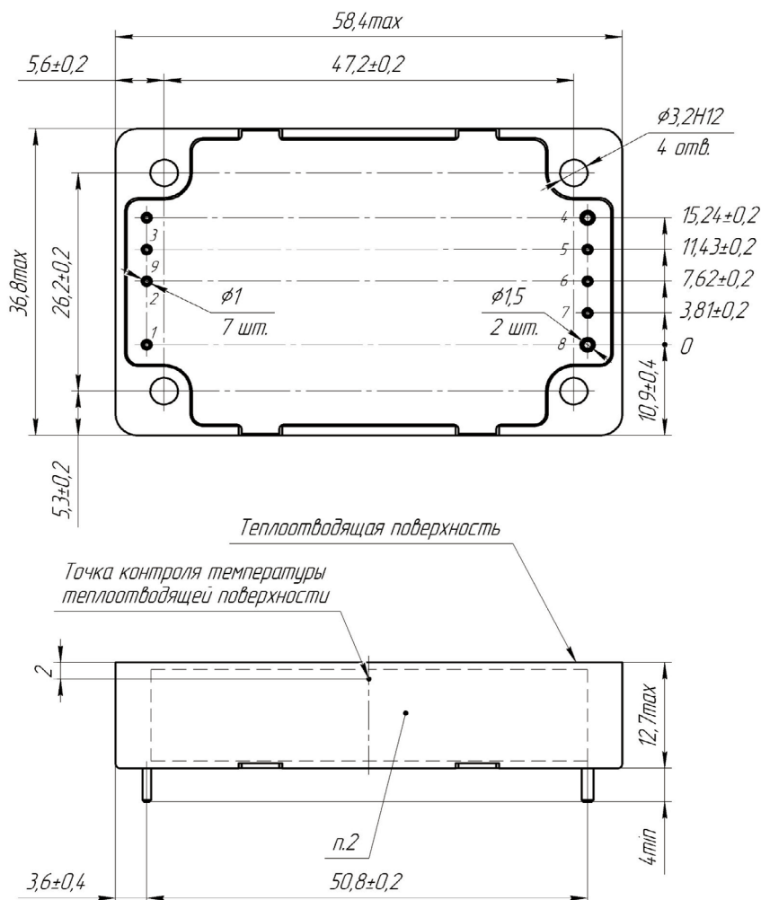
Рис. 20. Исполнение МДМ200-С.
