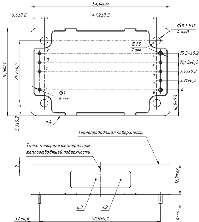
Рис. 1. Исполнение МДМ200-С.
