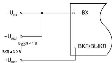
Рис. 5. Управление логическим напряжением.
