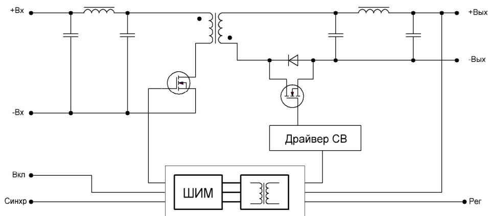
Рис. 1. Топология МДМ30-Б.
