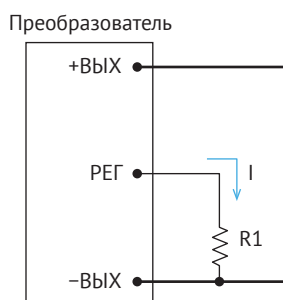
Рис. 9. Регулировка увеличением U_{\text{вых}} .
