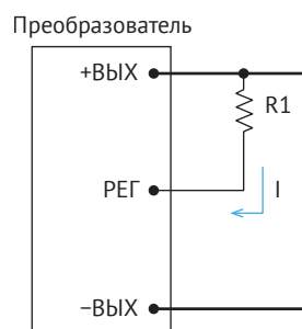
Рис. 10. Регулировка снижением U_{\text{вых}} .
