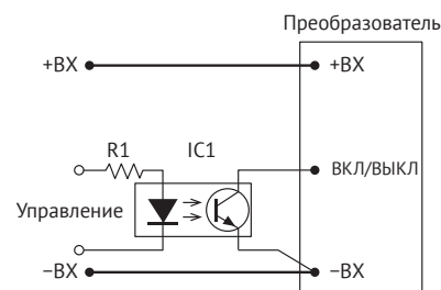
Рис. 8. «ДУ» с помощью оптрона.
