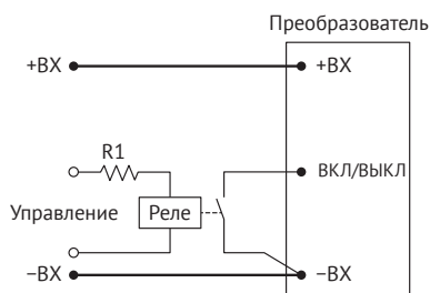
Рис. 6. «ДУ» с помощью реле.
