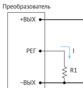
Рис. 7. Регулировка увеличением U_{VX} .
