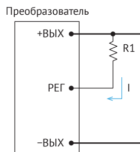
Рис. 8. Регулировка снижением U_{VX} .
