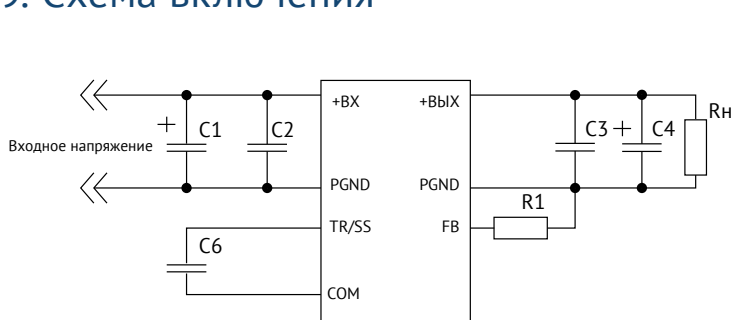
Рис. 3. Типовая схема включения модуля электропитания МНМ
