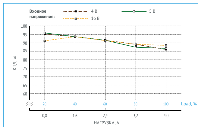
Рис. 20. КПД для МНМ4-1И1,05,0Т (U вых = 3,3 В).
