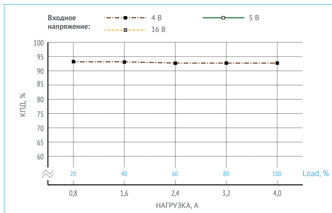
Рис. 21. КПД для МНМ4-1И1,05,0Т ( U_{\text{вых.}} = 5,0 \text{ В} ).
