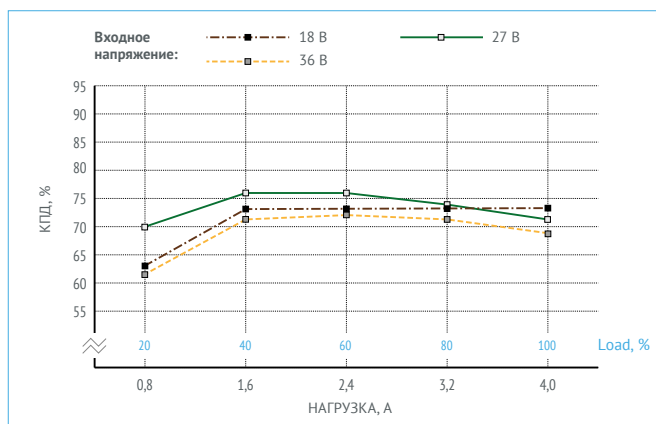
Рис. 8. КПД для МНМ4-1В1,05,0Т ( U_{\text{вых.}} = 1,0 \text{ В} ).
