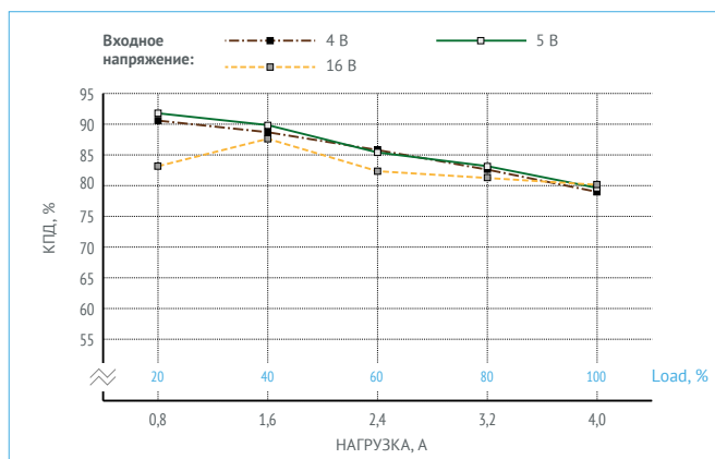
Рис. 17. КПД для МНМ4-1И1,05,0Т ( U_{\text{вых.}} = 1,5 \text{ В} ).
