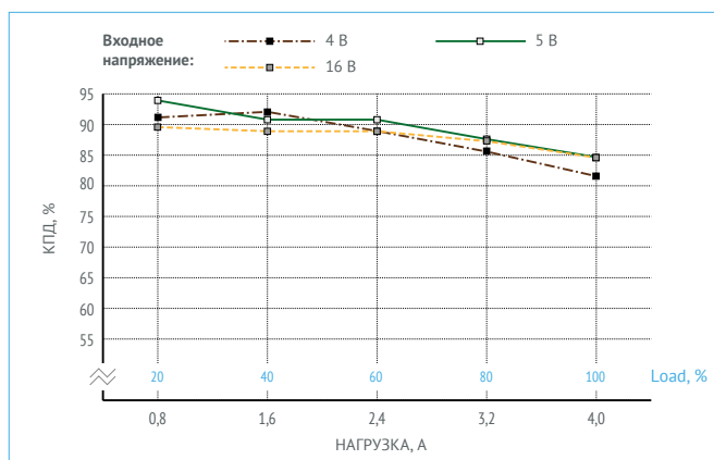
Рис. 19. КПД для МНМ4-1И1,05,0Т ( U_{\text{вых.}} = 2,5 \text{ В} ).
