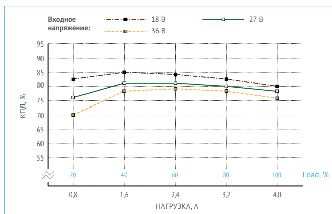
Рис. 10. КПД для МНМ4-1В1,05,0Т ( U_{\text{вых.}} = 1,5 \text{ В} ).
