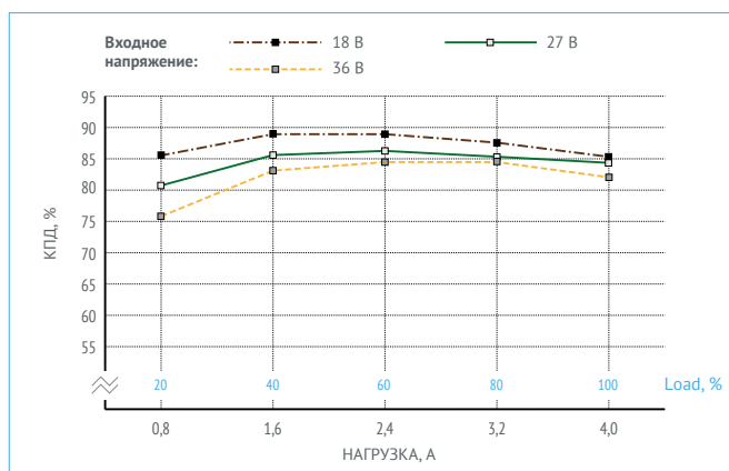
Рис. 12. КПД для МНМ4-1В1,05,0Т ( U_{\text{вых.}} = 2,5 \text{ В} ).
