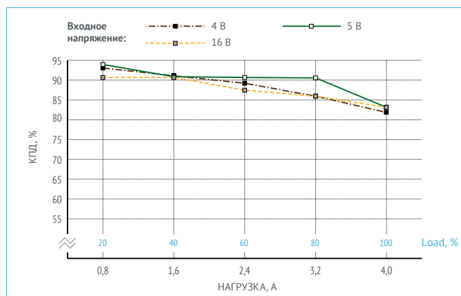
Рис. 18. КПД для МНМ4-1И1,05,0Т ( U_{\text{вых.}} = 2,0 \text{ В} ).
