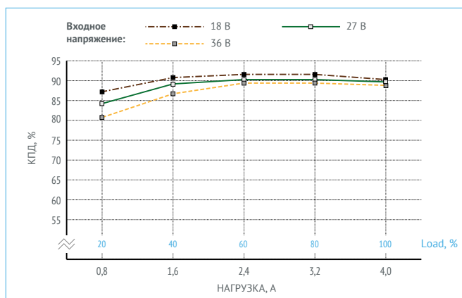
Рис. 14. КПД для МНМ4-1В1,05,0Т ( U_{\text{вых.}} = 5,0 \text{ В} ).
