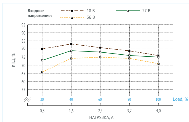
Рис. 9. КПД для МНМ4-1В1,05,0Т ( U_{\text{вых.}} = 1,2 \text{ В} ).
