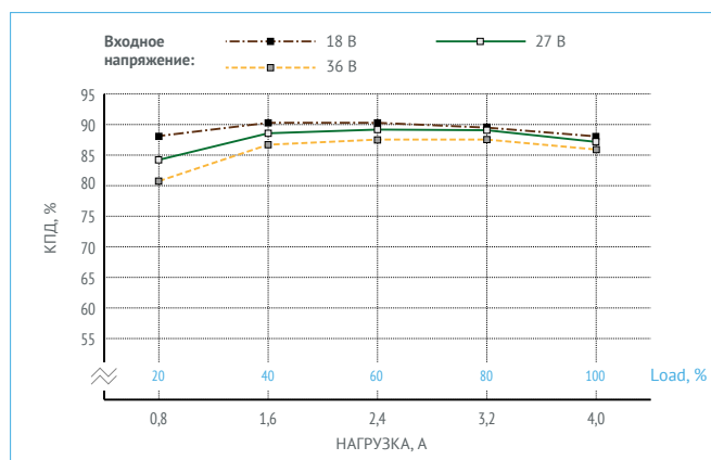
Рис. 13. КПД для МНМ4-1В1,05,0Т ( U_{\text{вых.}} = 3,3 \text{ В} ).
