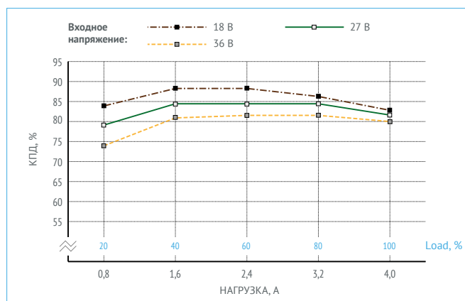
Рис. 11. КПД для МНМ4-1В1,05,0Т ( U_{\text{вых.}} = 2,0 \text{ В} ).
