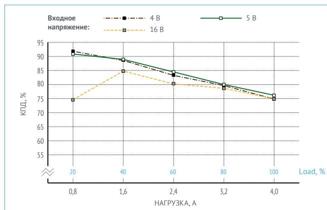
Рис. 16. КПД для МНМ4-1И1,05,0Т ( U_{\text{вых.}} = 1,2 \text{ В} ).
