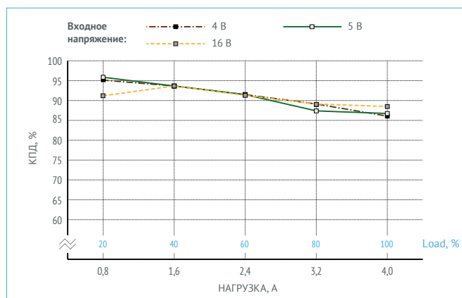
Рис. 20. КПД для МНМ4-1И1,05,0Т ( U_{\text{вых.}} = 3,3 \text{ В} ).
