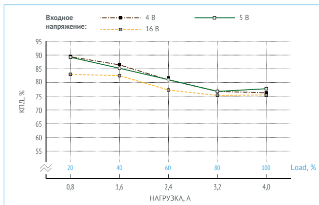
Рис. 15. КПД для МНМ4-1И1,05,0Т ( U_{\text{вых.}} = 1 \text{ В} ).
