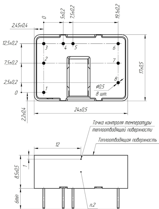
Рис. 12. Двухканальное исполнение.
