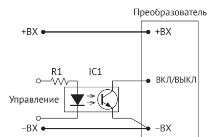
Рис. 7. «ДУ» с помощью оптрона.
