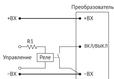
Рис. 5. «ДУ» с помощью реле.
