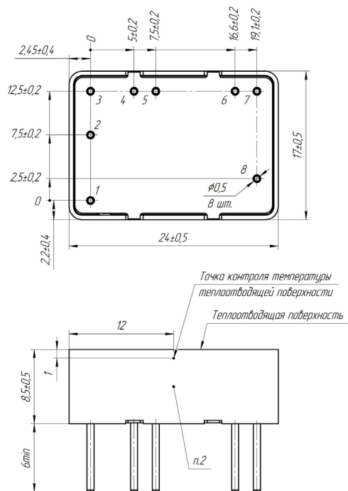
Рис. 11. Одноканальное исполнение.
