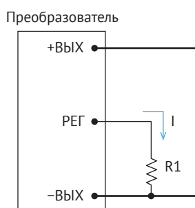
Рис. 8. Регулировка увеличением U_{\text{вых}} .
