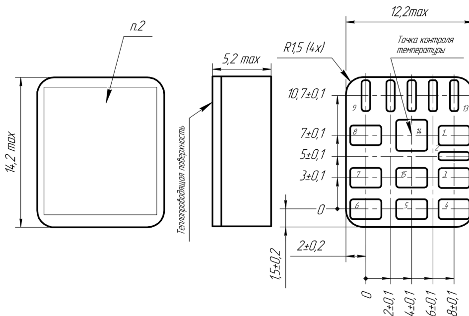
Рис. 6. Габаритный чертеж МНМ0,8.
