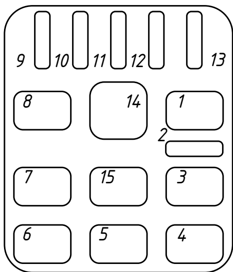
Рис. 1. Расположение контактных площадок модуля МНМО,8. Вид сверху.
