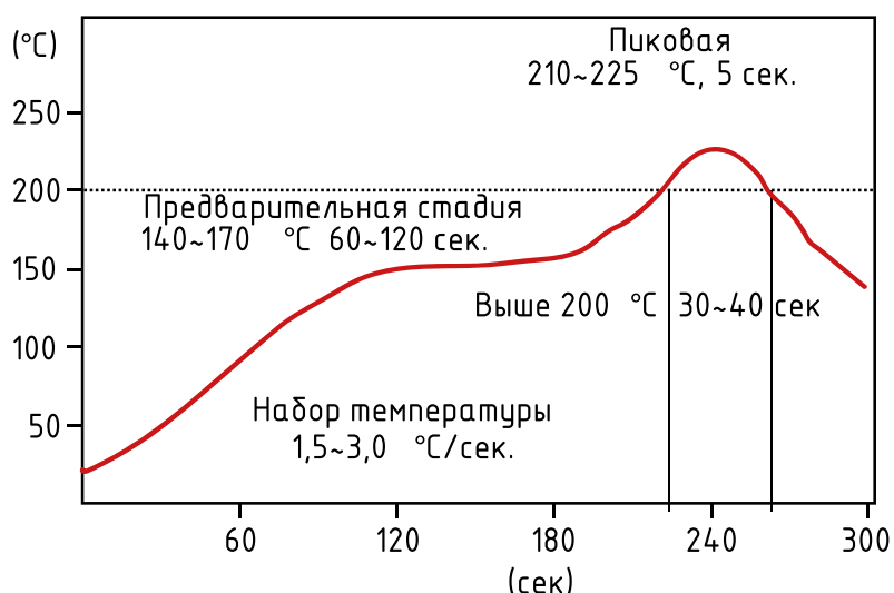
Рис. 4. Профиль оплавления.
