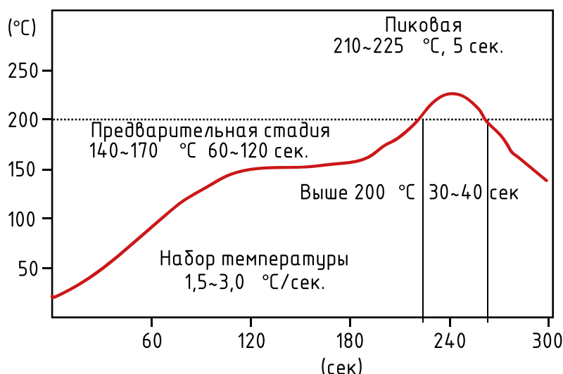
Рис. 5. Профиль оплавления.
