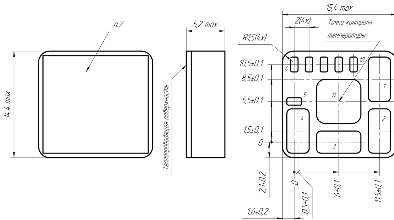
Рис. 7. Габаритный чертеж МНМ4.
