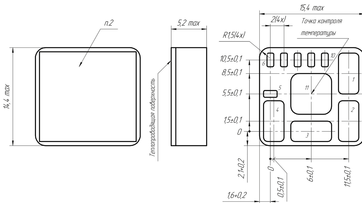
Рис. 7. Габаритный чертеж МНМ4.
