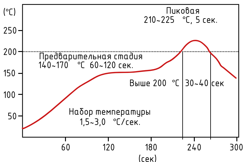
Рис. 5. Профиль оплавления.
