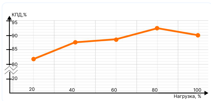
Рис. 8. КПД для МНМ4 (Выходное напряжение -12 В, входное напряжение 24 В)
