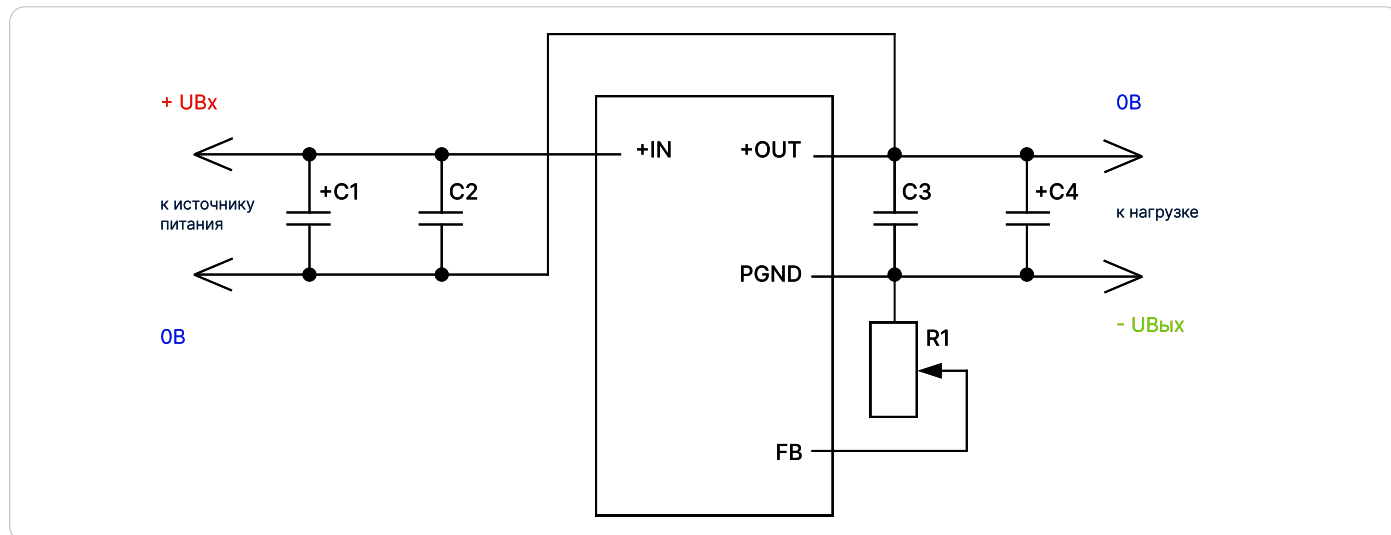
Рис. 3. Функциональная схема модуля МНМ для получения отрицательного U_{вых}
