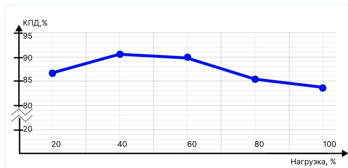
Рис. 10. КПД для МНМ4 (Выходное напряжение -15 В, входное напряжение 18 В)
