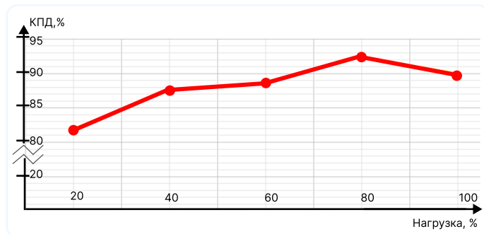
Рис. 9. КПД для МНМ4 (Выходное напряжение -9 В, входное напряжение 27 В)
