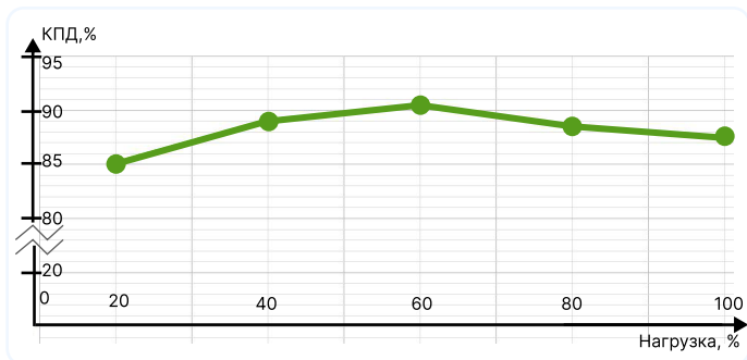
Рис. 7. КПД для МНМ4 (Выходное напряжение -5 В, входное напряжение 27 В)
