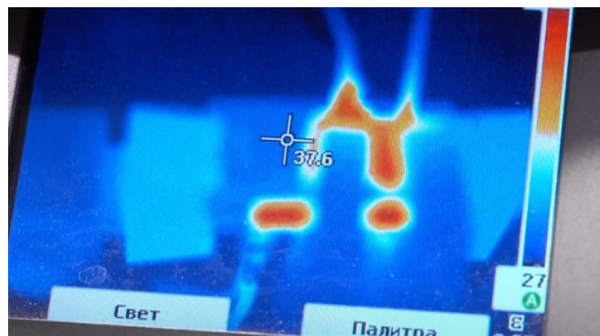
Рис. 11. Измерения T_{\text{корп}} для медного корпуса модуля с покрытием хим. никель. Бесконтактный метод - тепловизор.
