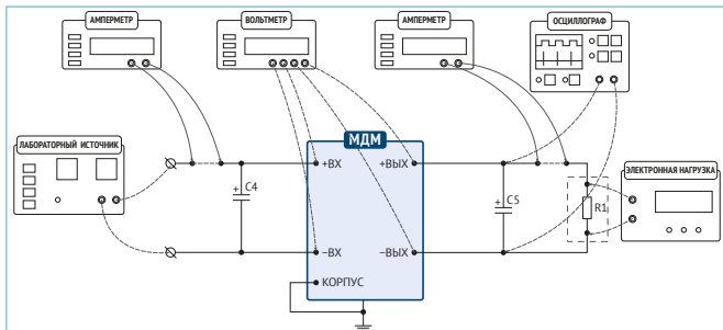
Рис. 8. Схема подключения оборудования и модуля.
