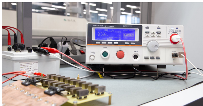
Стенд для проверки прочности изоляции
