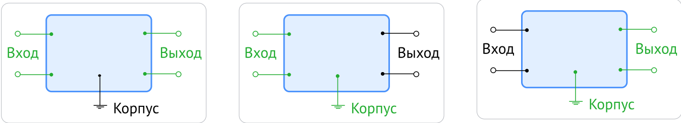
Рис. 1. Изоляция «Вход-Выход» Рис. 2. Изоляция «Вход-Корпус» Рис. 3. Изоляция «Выход-Корпус»
