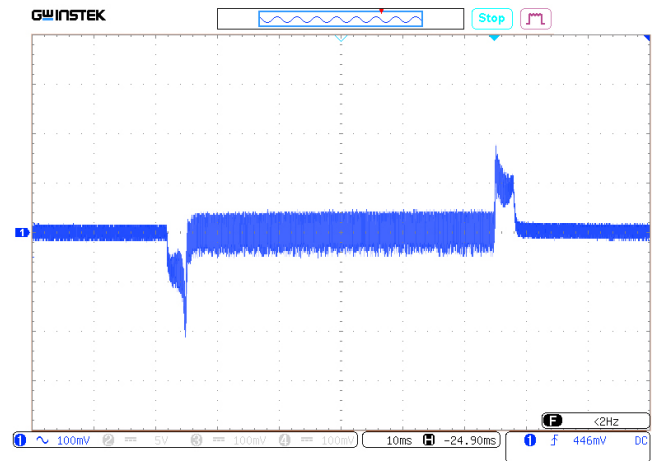
Рис. 17. Осциллограмма переходного отклонения выходного напряжения при изменении выходного тока с 10% до 100%. Масштаб 100 мВ/дел. Развертка 10 мс/дел.
