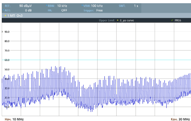
Рис. 31. Диапазон 10..30 МГц.
