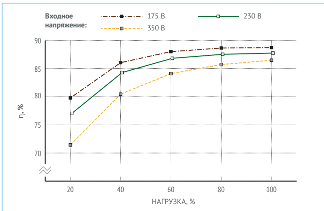
Рис. 13. МДМ160-1М27ТУП.
