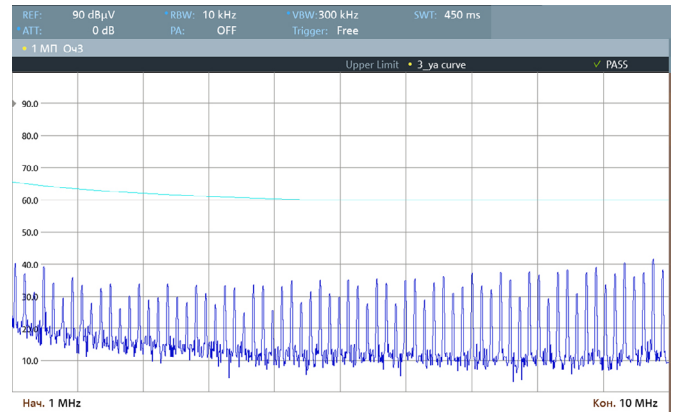
Рис. 34. Диапазон 1..10 МГц.
