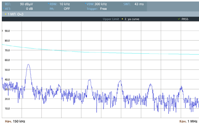
Рис. 33. Диапазон 0,15..1 МГц.
