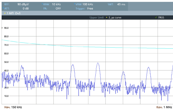
Рис. 25. Диапазон 0,15..1 МГц.
