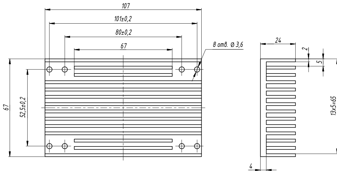
Рис. 40. БКЯЮ.752695.265-01.
