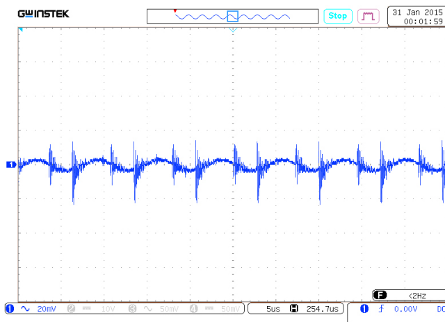
Рис. 24. Осциллограмма пульсаций выходного напряжения. Масштаб 20 мВ/дел. Развертка 5 мкс/дел.
