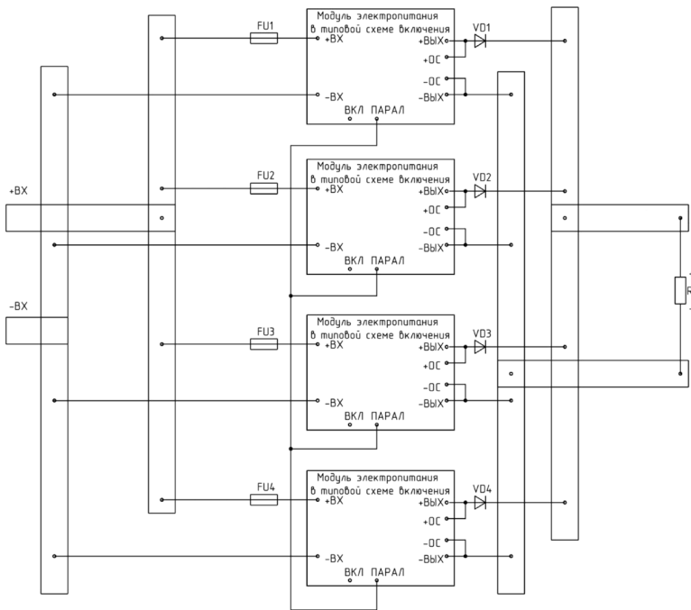
Рис. 8. Схема подключения модулей электропитания для параллельной работы (без указания элементов типовой схемы подключения [Рис. 2]).
