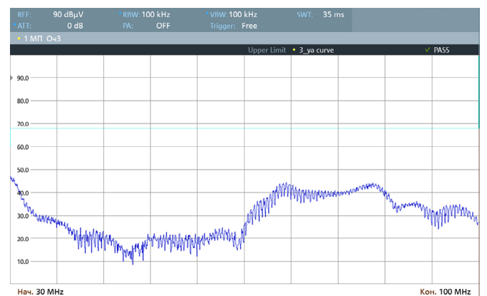
Рис. 32. Диапазон 30..100 МГц.
