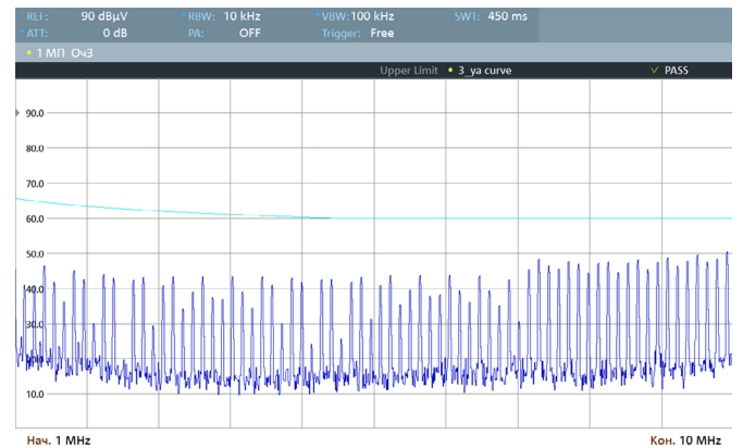
Рис. 26. Диапазон 1..10 МГц.
