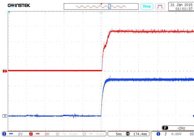
Рис. 22. Осциллограмма установления выходного напряжения с момента подачи команды дистанционного управления. Луч 1 (синий) – напряжение на выводе «ВКЛ». Масштаб 2 В/дел. Луч 2 (красный) – выходное напряжение. Масштаб 2 В/дел. Развертка 5 мс/дел.
