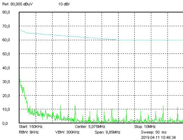
Рис. 40. Диапазон 0,15..10 МГц.
