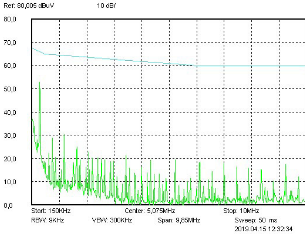
Рис. 38. Диапазон 0,15..10 МГц.
