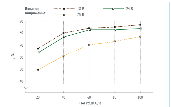
Рис. 22. МДМ50-1Ш12ТУР.
