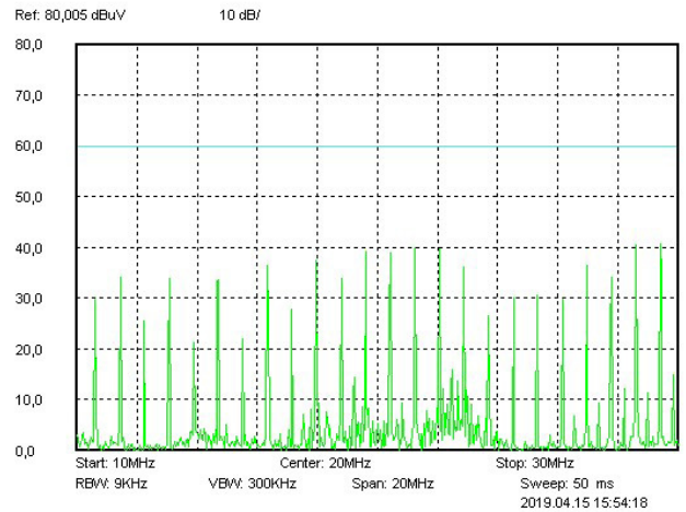
Рис. 41. Диапазон 10..30 МГц.
