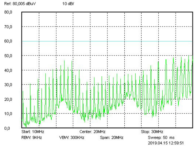
Рис. 39. Диапазон 10..30 МГц.
