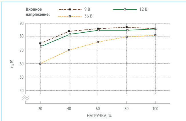
Рис. 18. МДМ50-1Б27ТУР.
