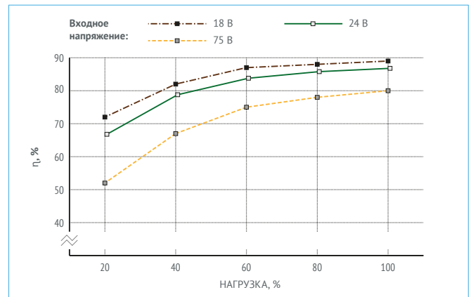
Рис. 20. МДМ50-1Ш05ТУР.
