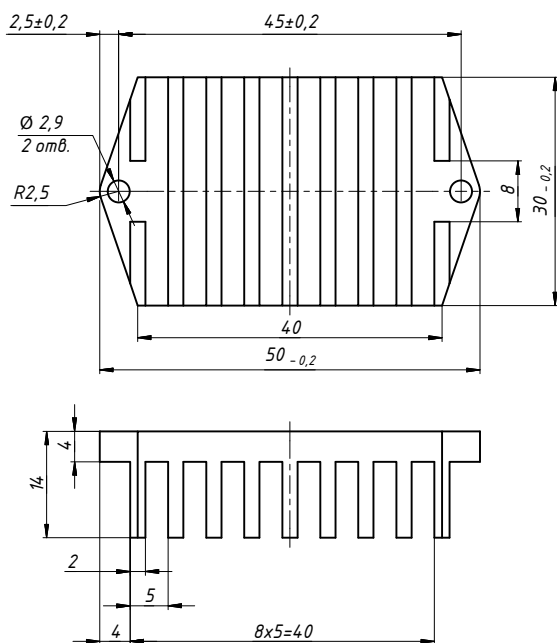
Рис. 43. БКЯЮ.752695.033.
