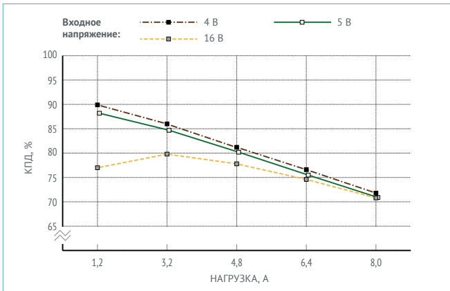
Рис. 15. КПД для МММ8-1И1,05,0Т. (Выходное напряжение 1 В).
