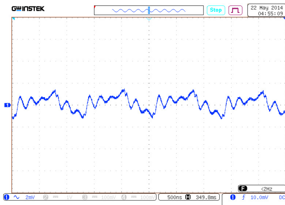
Рис. 31. Осциллограмма пульсаций выходного напряжения модуля при I_{OUT} = max . Масштаб 2 мВ/дел. Развертка 500 нс/дел.
