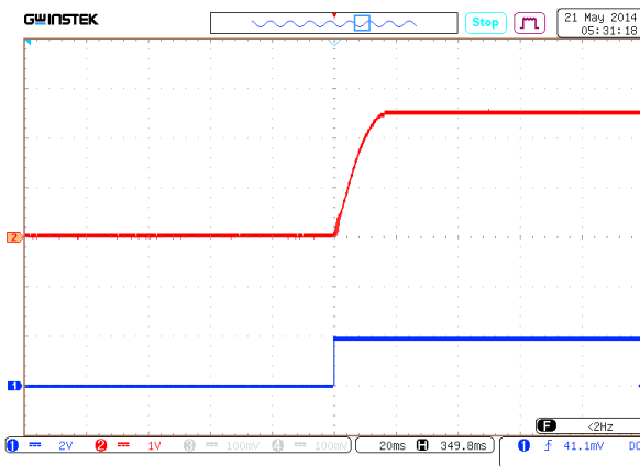
Рис. 22. Осциллограмма установления выходного напряжения с момента подачи команды дистанционного управления.
