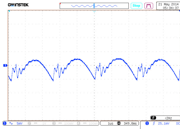
Рис. 26. Осциллограмма пульсаций выходного напряжения модуля Масштаб 5 мВ/дел. Развертка 1 мкс/дел.
