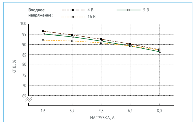
Рис. 20. КПД для МММ8-1И1,05,0Т. (Выходное напряжение 3,3 В).
