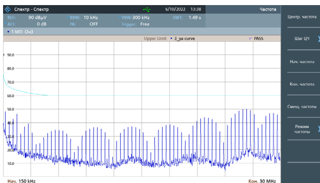
Рис. 32. Диапазон 0,15–30 MHz.
