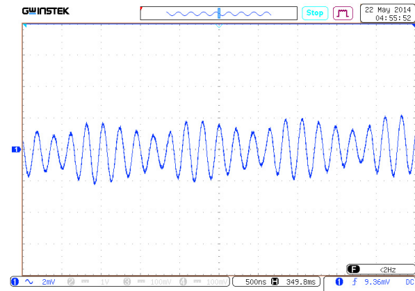
Рис. 30. Осциллограмма пульсаций выходного напряжения модуля в режиме пропуска импульсов.
