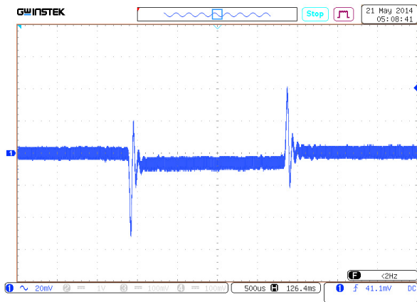
Рис. 24. Осциллограмма переходного отклонения выходного напряжения при изменении выходного тока. Масштаб 20 мВ/дел. Развертка 500 мкс/дел.
