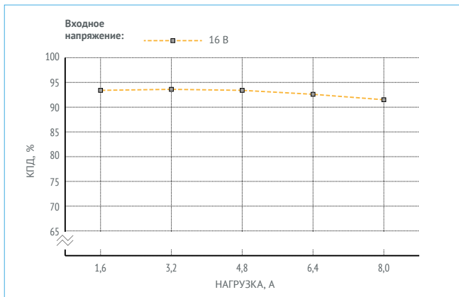
Рис. 21. КПД для МНМ8-1И05,0Т.
