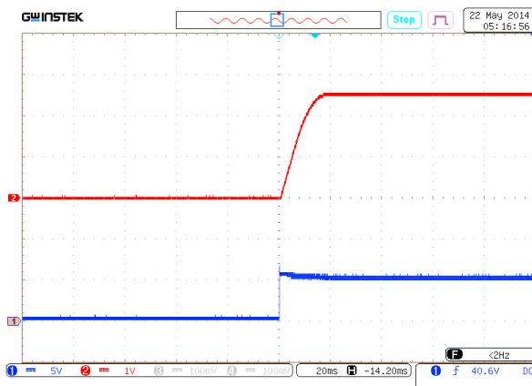
Рис. 28. Осциллограмма установления выходного напряжения с момента подачи входного напряжения.
