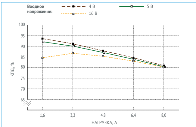
Рис. 18. КПД для МММ8-1И1,05,0Т. (Выходное напряжение 1,8 В).
