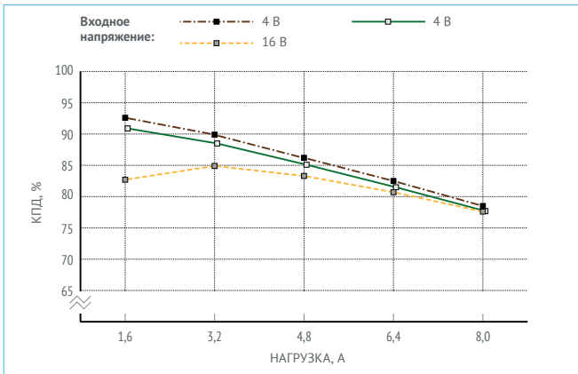
Рис. 17. КПД для МММ8-1И1,05,0Т. (Выходное напряжение 1,5 В).
