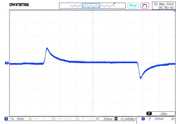
Рис. 29. Осциллограмма переходного отклонения выходного напряжения при изменении выходного тока.
