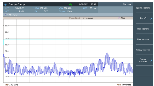
Рис. 33. Диапазон 30–100 MHz.
