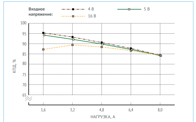
Рис. 19. КПД для МММ8-1И1,05,0Т. (Выходное напряжение 2,5 В).
