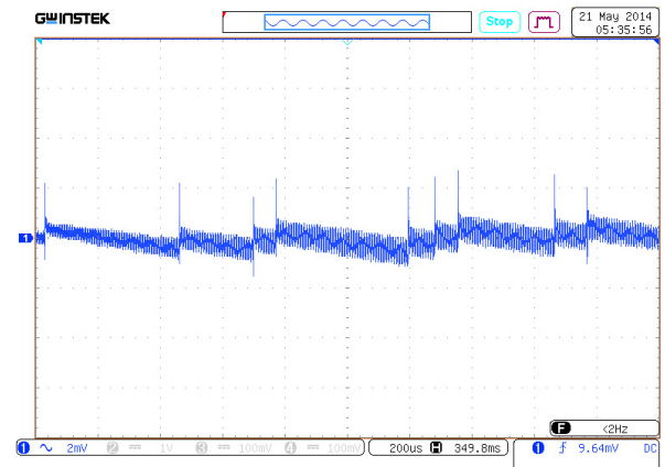
Рис. 25. Осциллограмма пульсаций выходного напряжения модуля в режиме пропуска импульсов. Масштаб 2 мВ/дел. Развертка 200 мкс/дел. I_{\text{ВЫХ}} = 0\text{А} .
