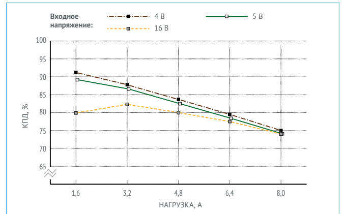
Рис. 16. КПД для МММ8-1И1,05,0Т. (Выходное напряжение 1,2 В).
