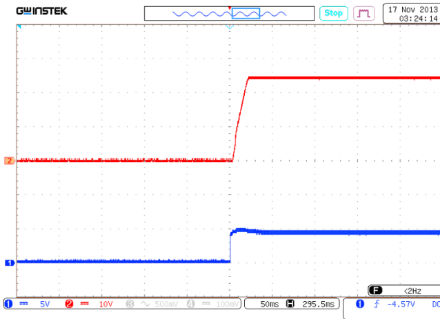
Рис. 31. Осциллограмма установления выходного напряжения с момента подачи команды дистанционного управления. Луч 1 (синий) – напряжение на выводе «VKЛ». Масштаб 5 В/дел. Луч 2 (красный) – выходное напряжение. Масштаб 10 В/дел. Развертка 50 мс/дел.
