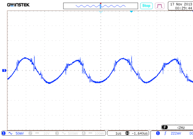
Рис. 33. Осциллограмма пульсаций выходного напряжения. Масштаб 50 мВ/дел. Развертка 1 мкс/дел.
