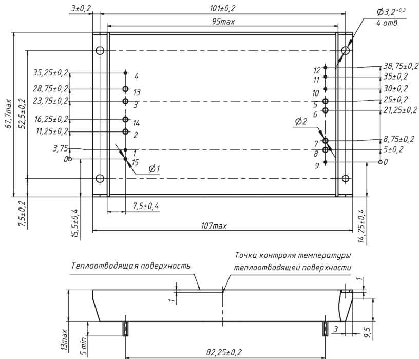
Рис. 37. Исполнение в усиленном корпусе с фланцами для МДМ400-Р, МДМ500-Р.
