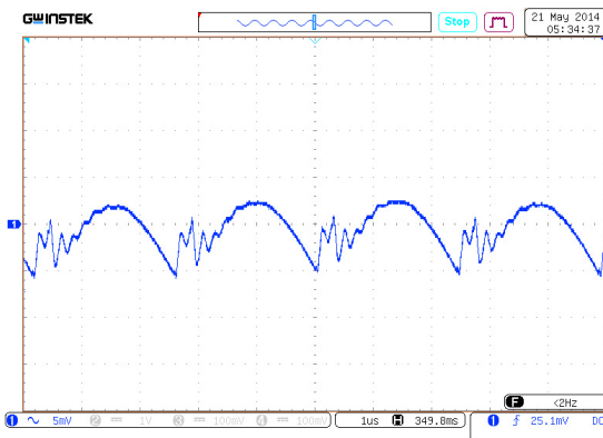
Рис. 10. Осциллограмма пульсаций выходного напряжения модуля при I_{OUT} = 8\text{ A} . Масштаб 5 мВ/дел. Развертка 1 мкс/дел.
