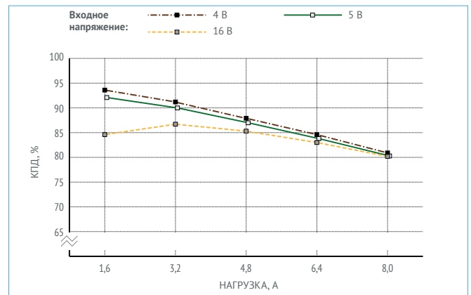
Рис. 29. КПД для МНМ8-1И1,05,0Т. (Выходное напряжение 1,8 В).
