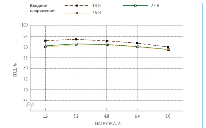
Рис. 24. КПД для МНМ8-1В1,05,0Т. (Выходное напряжение 5 В).
