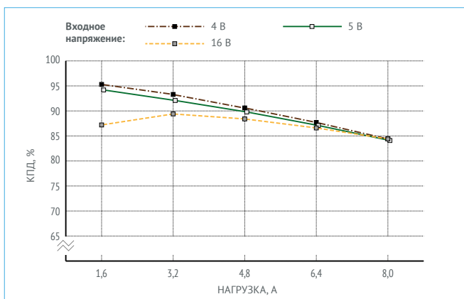
Рис. 28. КПД для МНМ8-1И1,05,0Т. (Выходное напряжение 2,5 В).
